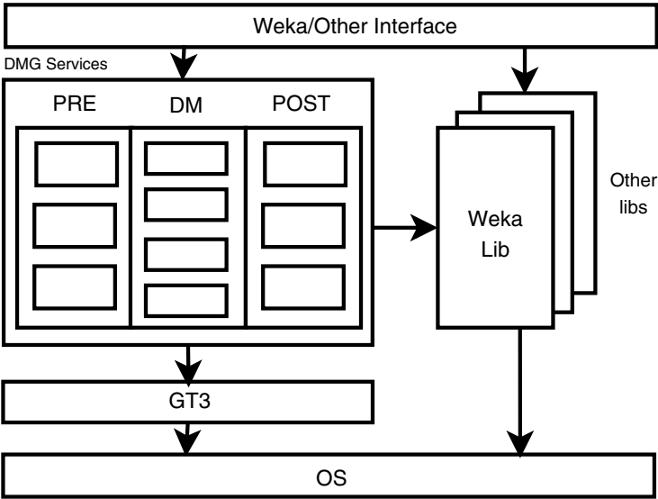
Fig. 1. DMGA Overview
